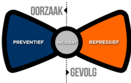
Figuur 7: Vlinderdasmodel
